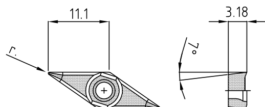
VCGT..N-Alu-FA-G7B
