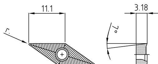
VCGT..N-Alu-FB-G7B
