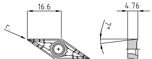
VCGT..N-AWI-FA-G7B
