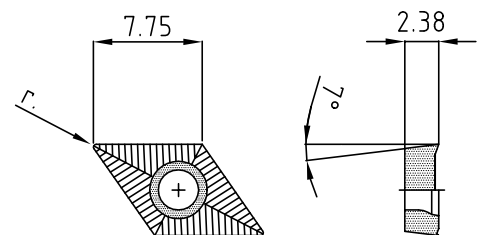
DCGT..N-Alu-FB-G7B
