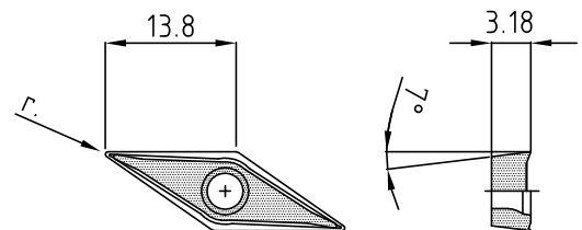
VCGT..N-ASF-FA
