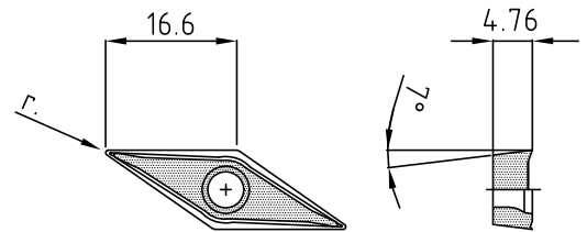
VCGT..N-ASF-FA
